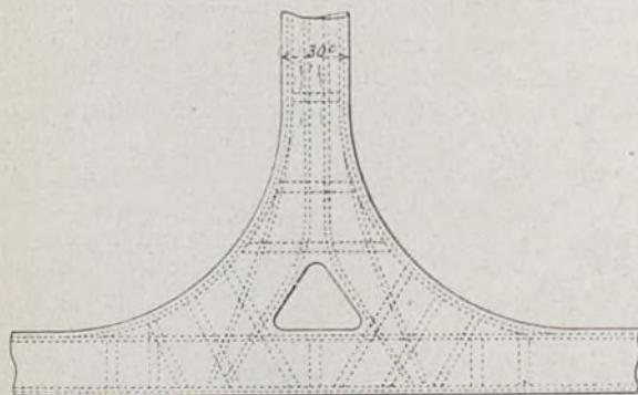
Fig. 2. Unión de un montante con la cabeza inferior.
