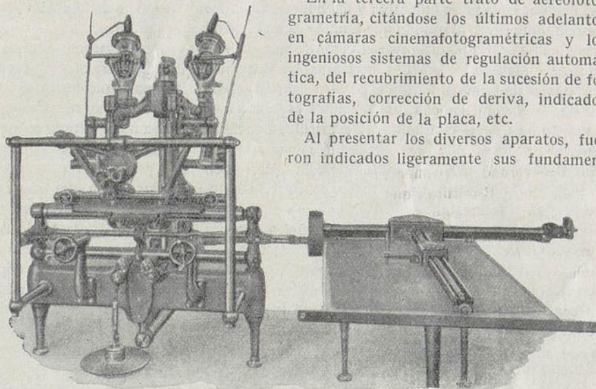
El Estereoplanígrafo ZEISS
