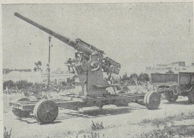
Cañón antiaéreo del crucero «Almirante Cervera».
