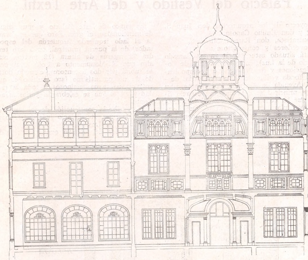
Casa de la Prensa. Sección B. E. 1/50.
