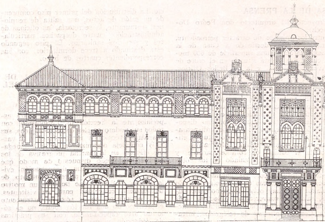
Casa de la Prensa. Fachada, Avenida del Marqués de Comillas. E. 1/50.
