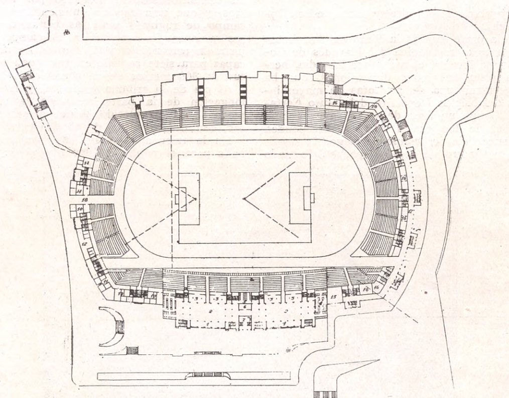
ESTADIO DE LA EXPOSICION DE BARCELONA. — Planta baja. Escala 1/1000
