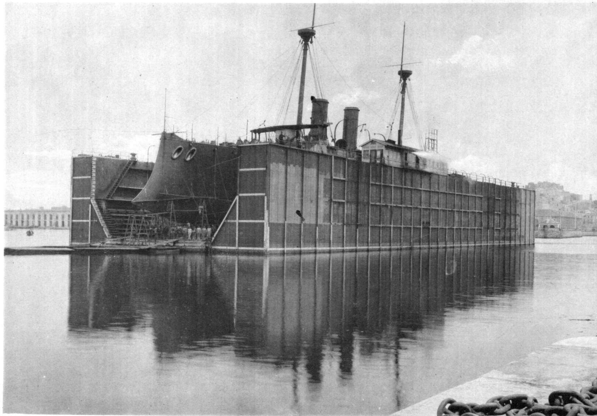
EL CRUCERO «LEPANTO» EN EL DIQUE FLOTANTE
