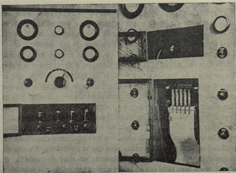
En la central de relojes hay también una instalación receptora de las señales horarias de Nauen. Las señales se reciben por una antena del receptor conectado a la red.
