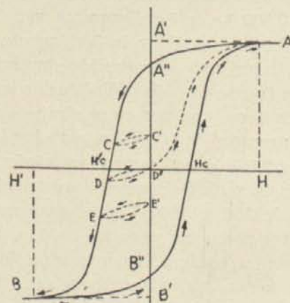
Figura 1. a Ciclo de histéresis magnética en el que se funda el procedimiento de impresión y reproducción magnética del sonido.
