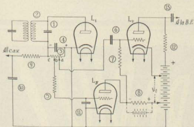
riente de placa, que hasta puede llegar a ser nula, en cuyo caso no se producirá caída alguna en (8), lo que equivale a suprimir la pila figurada y, por tanto, la lámpara L_2 quedará a una polarización -V_K normal para el buen funcionamiento de la misma. Así, pues, las señales potentes se podrán oír bien, ya que su acción respecto a L_5 deja a L_2 en condiciones perfectas de polarización.
