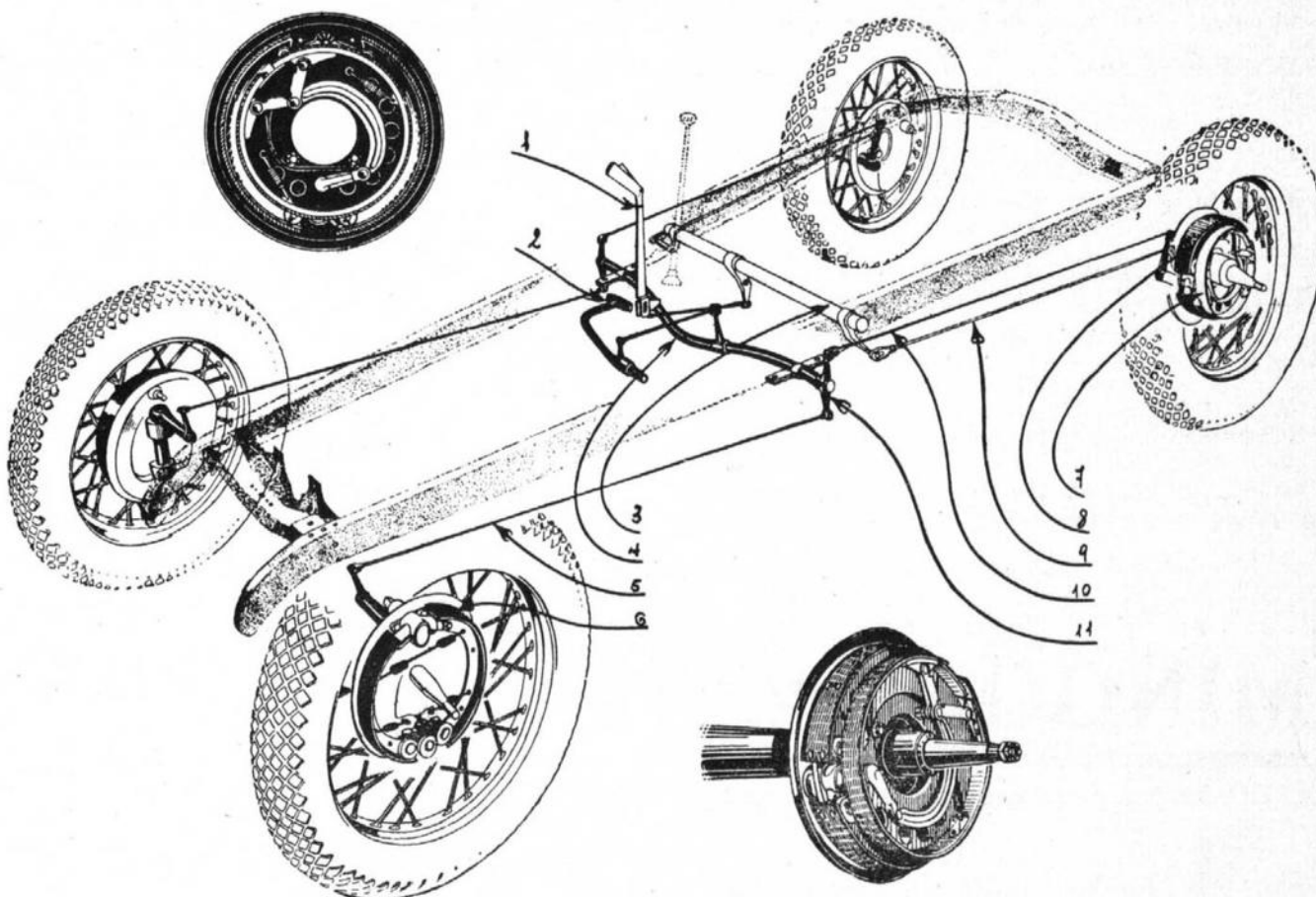
1, Palanca de freno de mano; 2, Pedal de mando de los frenos sobre las cuatro ruedas; 3, Arbol transversal del freno de mano; 4, Arbol de mando de los frenos sobre las cuatro ruedas; 5, Varilla de mando del freno de mano; 6, Mordaza de freno delantero; 7, Mordaza de freno de mano trasero; 8, Mordaza de freno de pie trasero; 9, Varilla de mando del freno de mano; 10, Varilla de mando del freno de pie trasero; 11, Balancín que equilibra los frenos delanteros y traseros.
