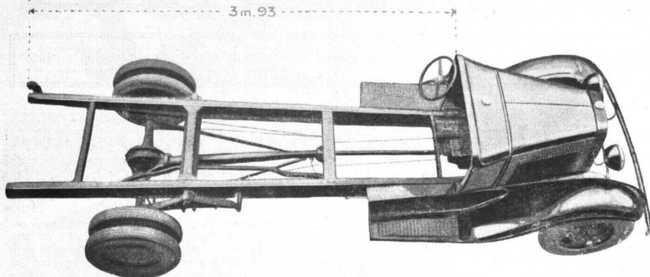
El nuevo chasis largo. (Obsérvese que la longitud desde el tablero al extremo del chasis para colocar la carrocería es de 3,93 metros.)
