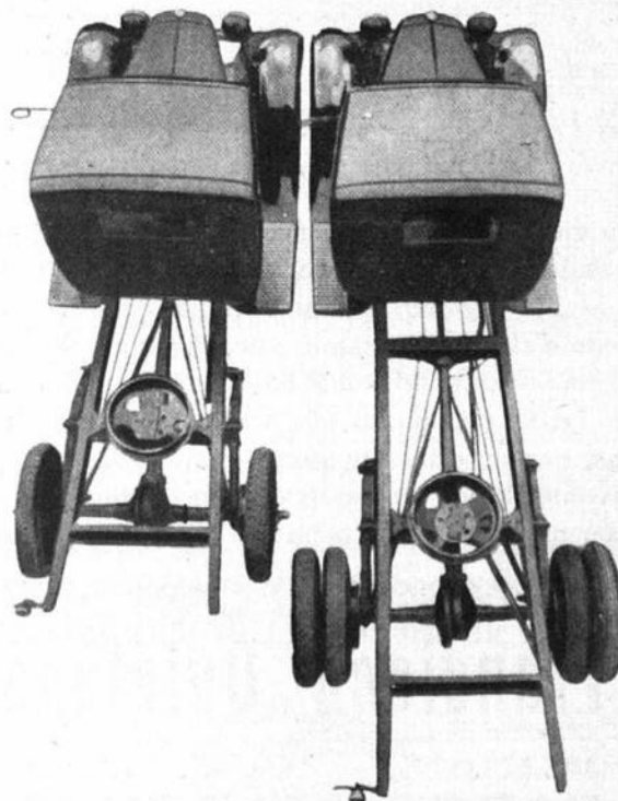
Fotografía comparativa del chasis normal y del chasis largo
