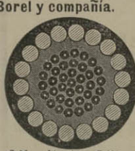
Cable subterráneo, Teléfono múltiplo.
