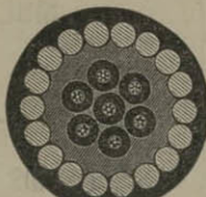
Cable submarino múltiplo.
