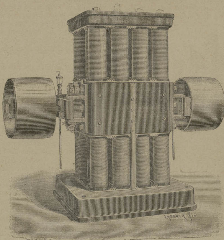
FIG. 14.—Máquina Gramme.
