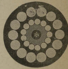
Cable submarino.
