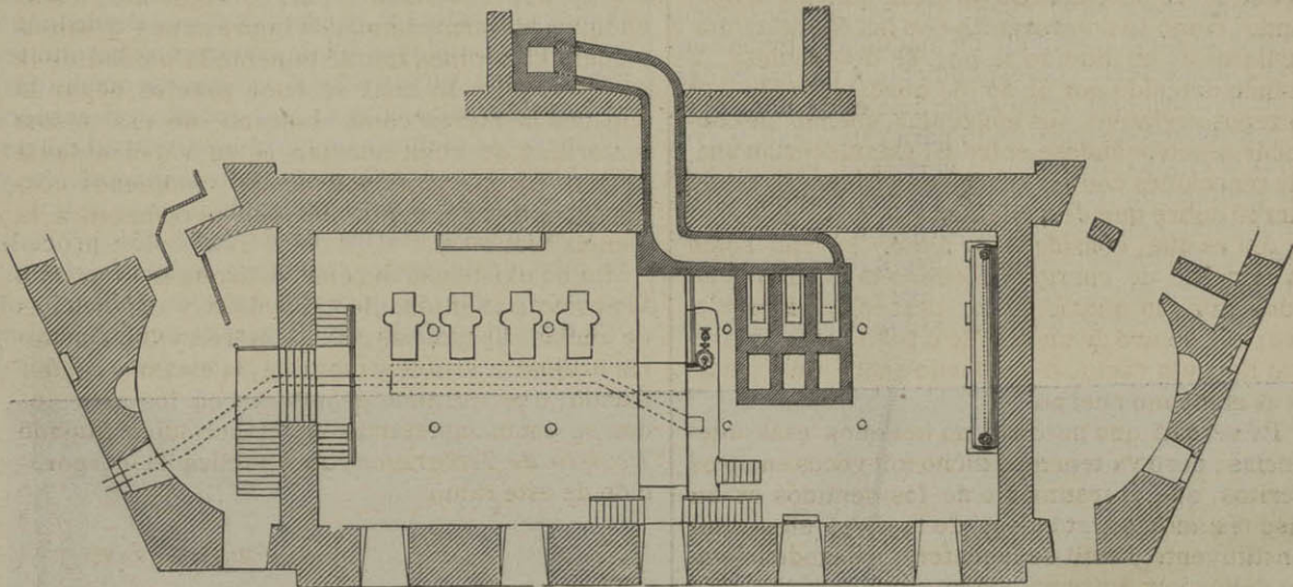
FIG. 20. —Planta general de los departamentos de máquinas y calderas.
