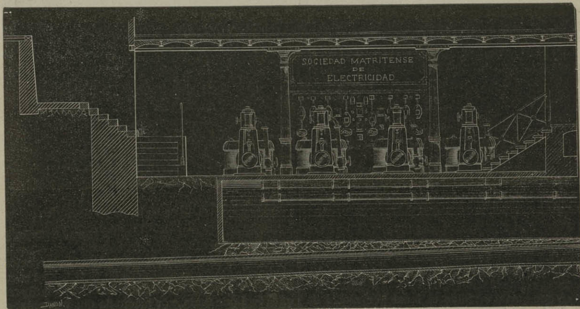
FIG. 21. —Perfil longitudinal del departamento de máquinas.
