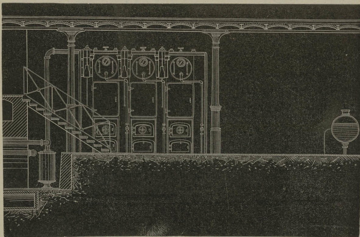
FIG. 22.—Perfil longitudinal del departamento de calderas.
