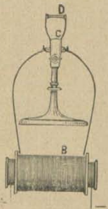
FIG. 2.—Vista exterior de las lámparas Nernst.
