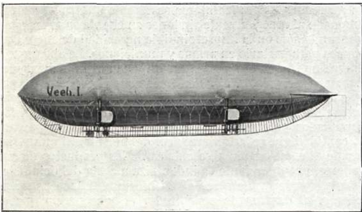
Dirigible alemán Veeh I , semirrígido, de 9,100 m. 3 ; longitud, 70 m.; diámetro, 12'4 m.; motores, 260 H. P.; velocidad, 70 kilóm. Construido 1911-13
