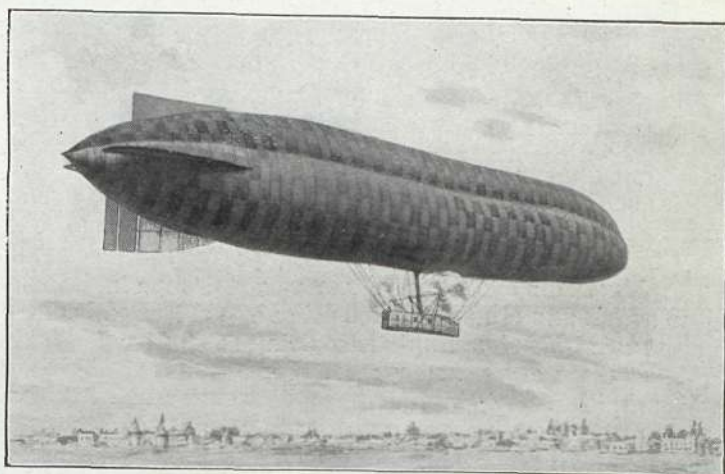
Dirigible inglés Astra Torres XIV , flexible, de 8,700 m. 3 ; longitud, 77 m.; diámetro, 18 m.; motores, 400 H. P.; velocidad, 82'2 kilóm. Construido en 1913
