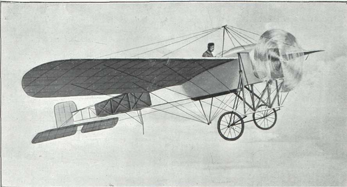
Monoplano francés Blériot , modelo 1913; peso, 355 kg.; motor Gnome de 80 caballos; velocidad, 115-120 kilóm.
