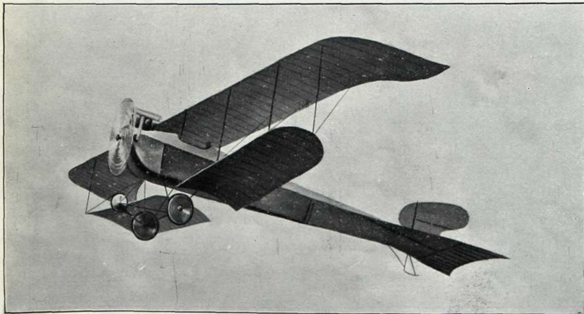
Biplano alemán A. E. G. , modelo 1913; motor N. A. G. de 100 caballos; velocidad, 90-100 kilóm.
