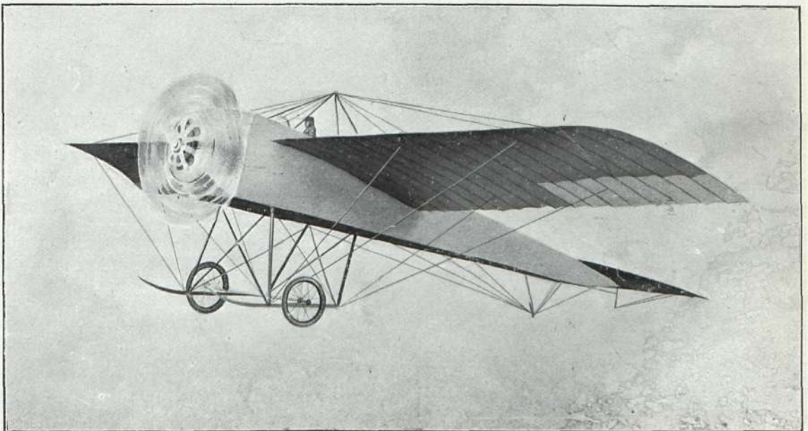
Monoplano francés Henry Farman , modelo 1913; peso, 285 kg.; motor Gnome de 50/80 caballos; velocidad, 105-110 kilóm.
