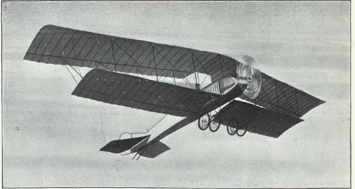
Biplano alemán Aviatik , modelo 1912-13; peso, 690 kg.; motor Argus-Mercedes de 100 caballos; velocidad, 100 kilóm.
