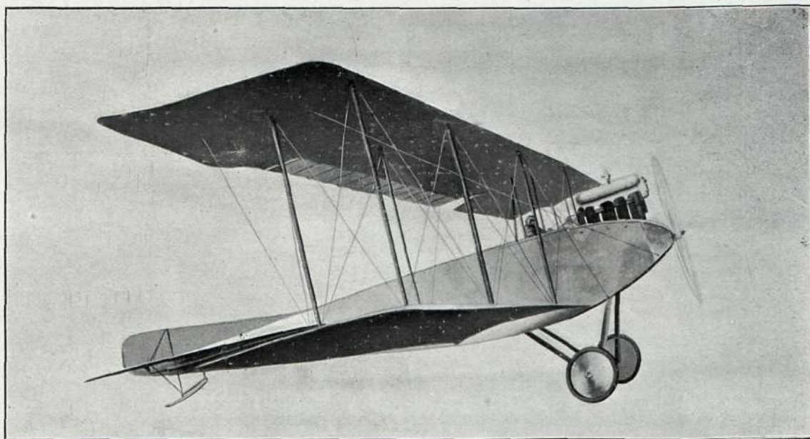
Biplano alemán Albatros , modelo 1913; peso, 620 kg.; motor Argus-Mercedes de 100 caballos; velocidad, 110 kilóm.
