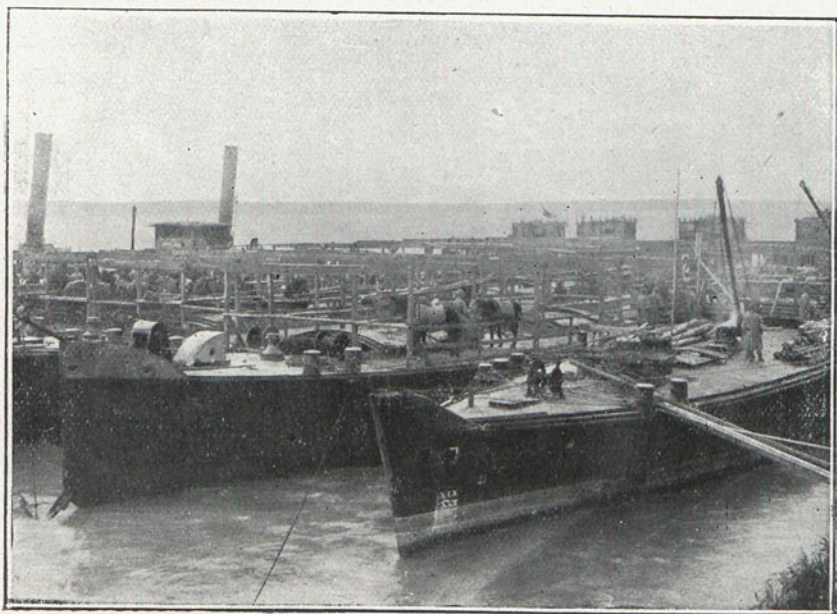
Barcazas para el paso del Danubio.
