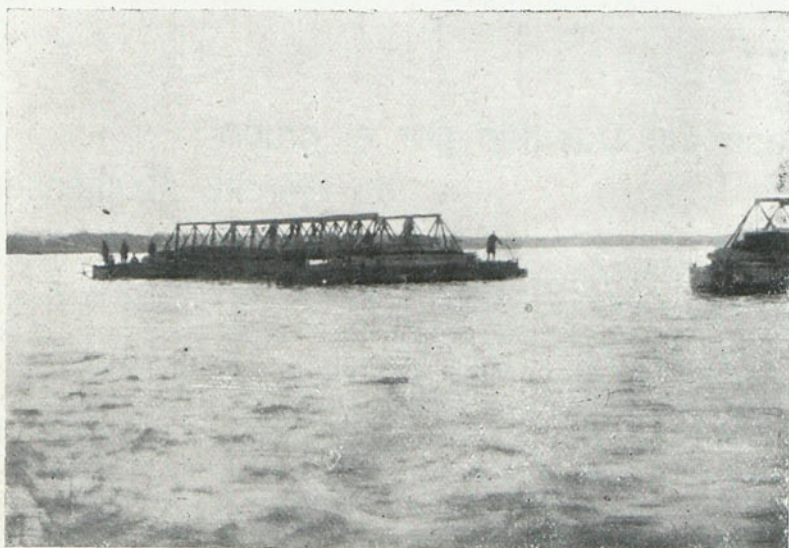
Construcción del puente cerca de Svistov.
