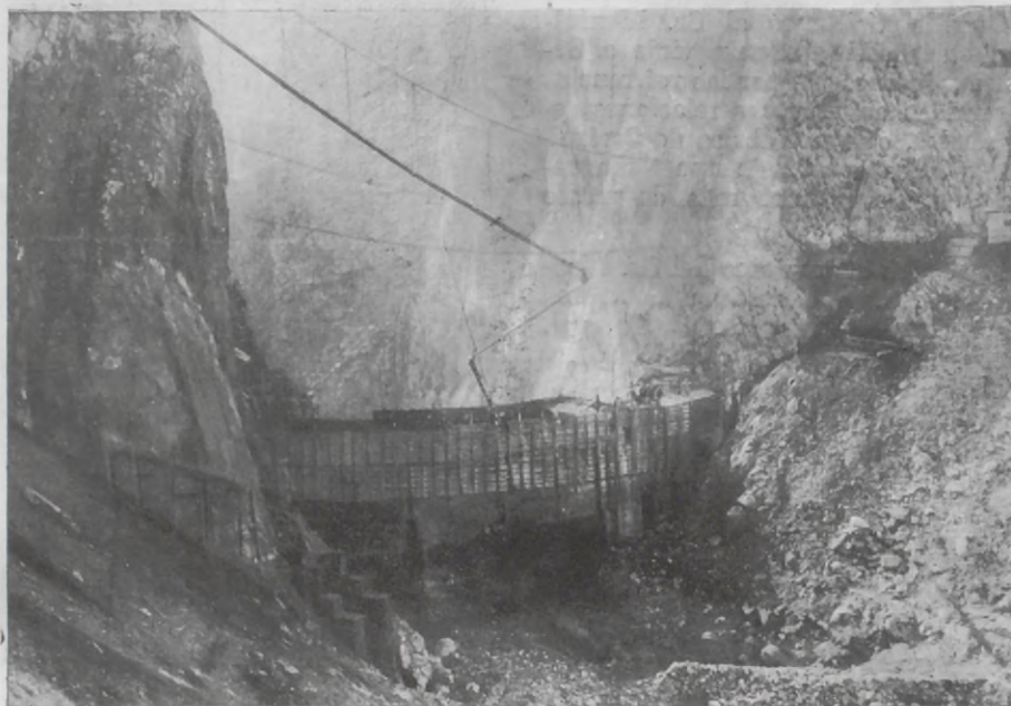
Central eléctrica y pàntano de Montejaque (en construcción en la provincia de Málaga), propiedad de la Compañía Sevillana de Electricidad.
