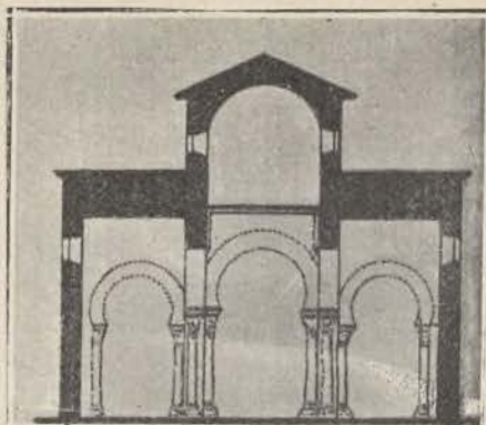
Lebeña. — Arcatura interna
