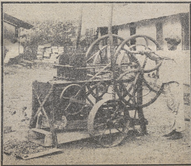
Descascaradora de cacao, inventada por el reverendísimo padre Coll. Fué premiada con medalla de oro en la Exposición de Calabar
