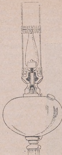
4 —LÁMPARA DE ALCÓHOL DE INCANDESCENCIA
