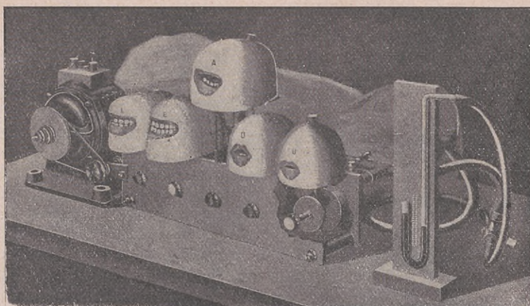
Fig. 12. —Aparatos de síntesis de las vocales
