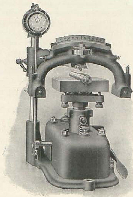
Péndulo con su sostén
