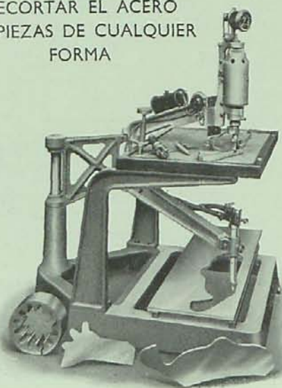
Maquina Perfiladora Num. 01 con movimiento automatico
