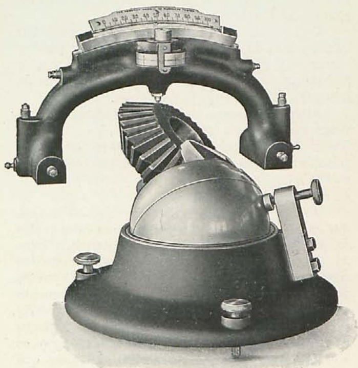
El Péndulo "Herbert"
