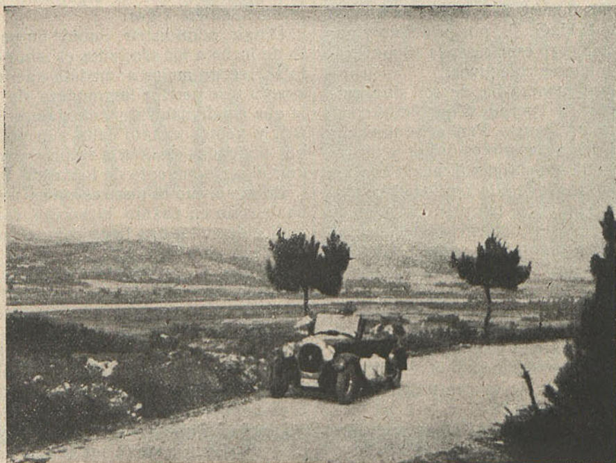
El río Ulla y la vega de Padrón y Cesures (Coruña).
