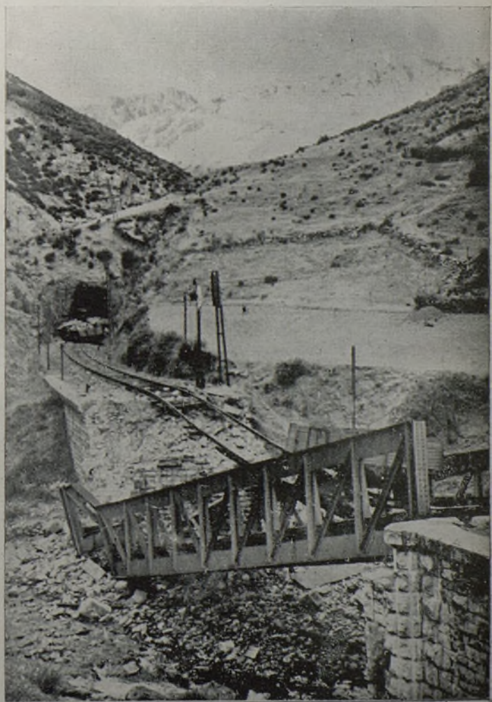
Frente de León: Puente volado, con un vagón de carbón sobre la vía.
