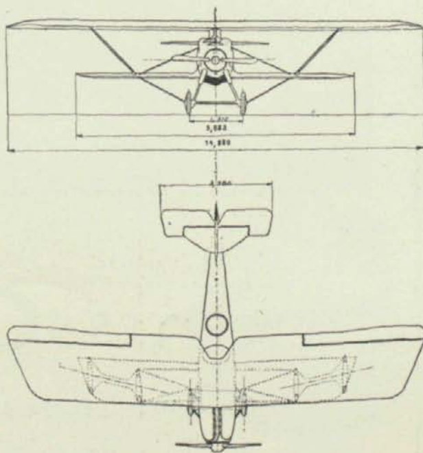
Vistas esquemáticas del sexquiplano.
