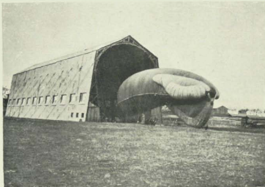
Entrada de un globo «Cacquot» en el hangar.
