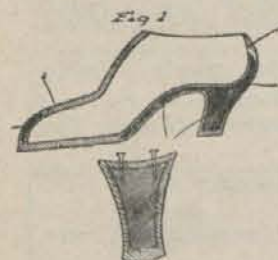
Tacón de goma con núcleo interior más duro, para sujetarle con tornillos.
