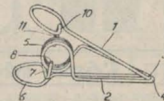
Pinza con muelle de una sola pieza.
