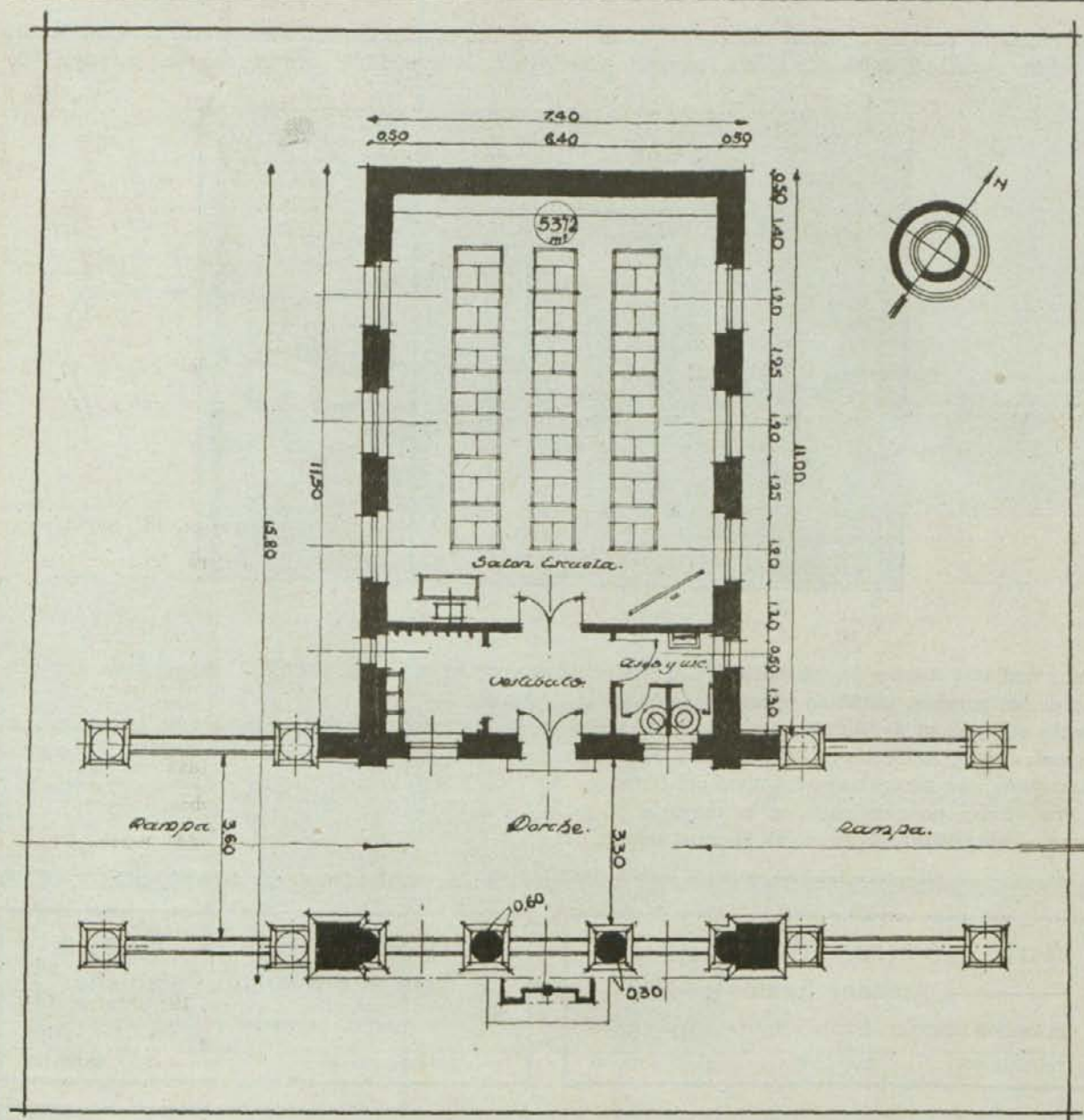
Plano de plantas. (Figura núm. 6.)
