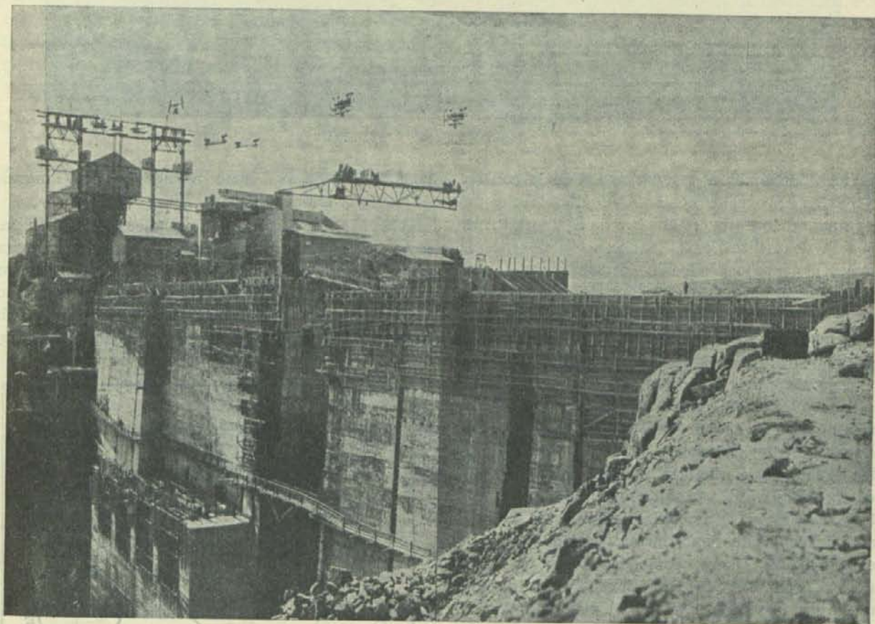
Presa del Esla.—En el centro del gigantesco muro próximo a terminarse, se ve el portillo por el que actualmente pasa el río y que se cerrará al finalizar la obra. Al fondo, las instalaciones para la fabricación y colocación de hormigón que han permitido levantar en menos de dos años este monolito de más de 350.000 metros cúbicos
