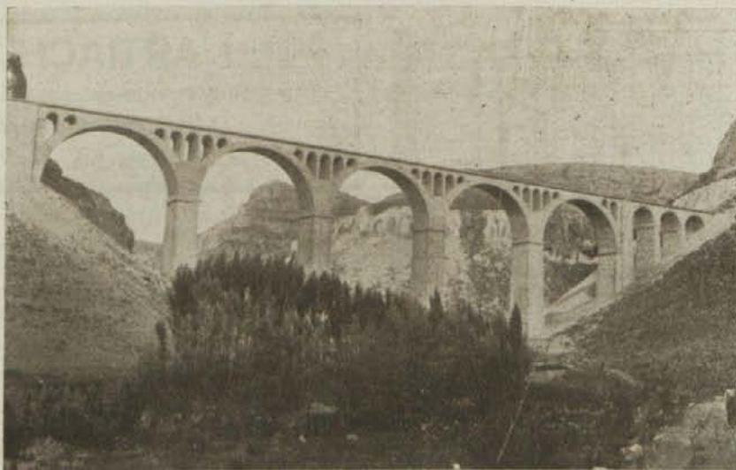
Obras del ferrocarril Madrid-Burgos.—El puente sobre el Riaza, en Linares del Arroyo, es una hermosa obra de la ingeniería. Tiene 50 metros de altura y será, quizás, la obra más atrevida del trazado
