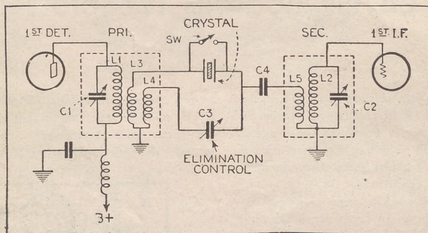
Fig. 4.—Circuit d'alta freqüència amb cristall
