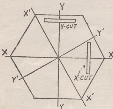
Fig. 1.—Secció d'un cristall de quars
