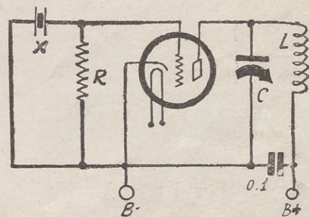
Fig. 2.—Cristall intercalat en el circuit de reixeta
