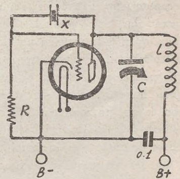
Fig. 3.—Cristall intercalat entre reixeta i placa
