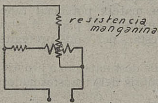
Amperímetre Fig. 29
