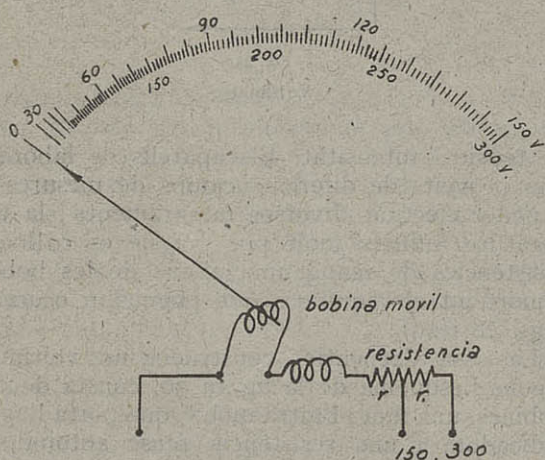
Voltímetre Fig. 30
