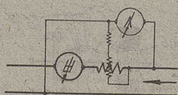
Fig. 24 Circuit de tensió abans del Voltímetre
