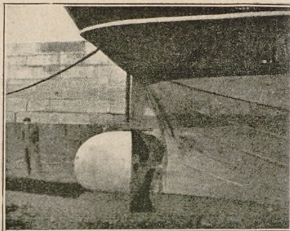
Fig. 5. Vista del timón Litehen aplicado a la embarcación de cabotaje Alca
