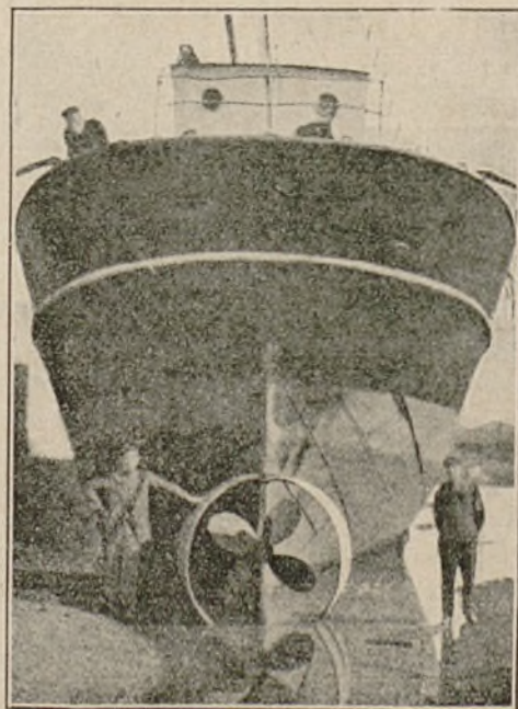
Fig. 6. Vista posterior del Alca
