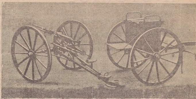
La Hotchkis con cureña.
