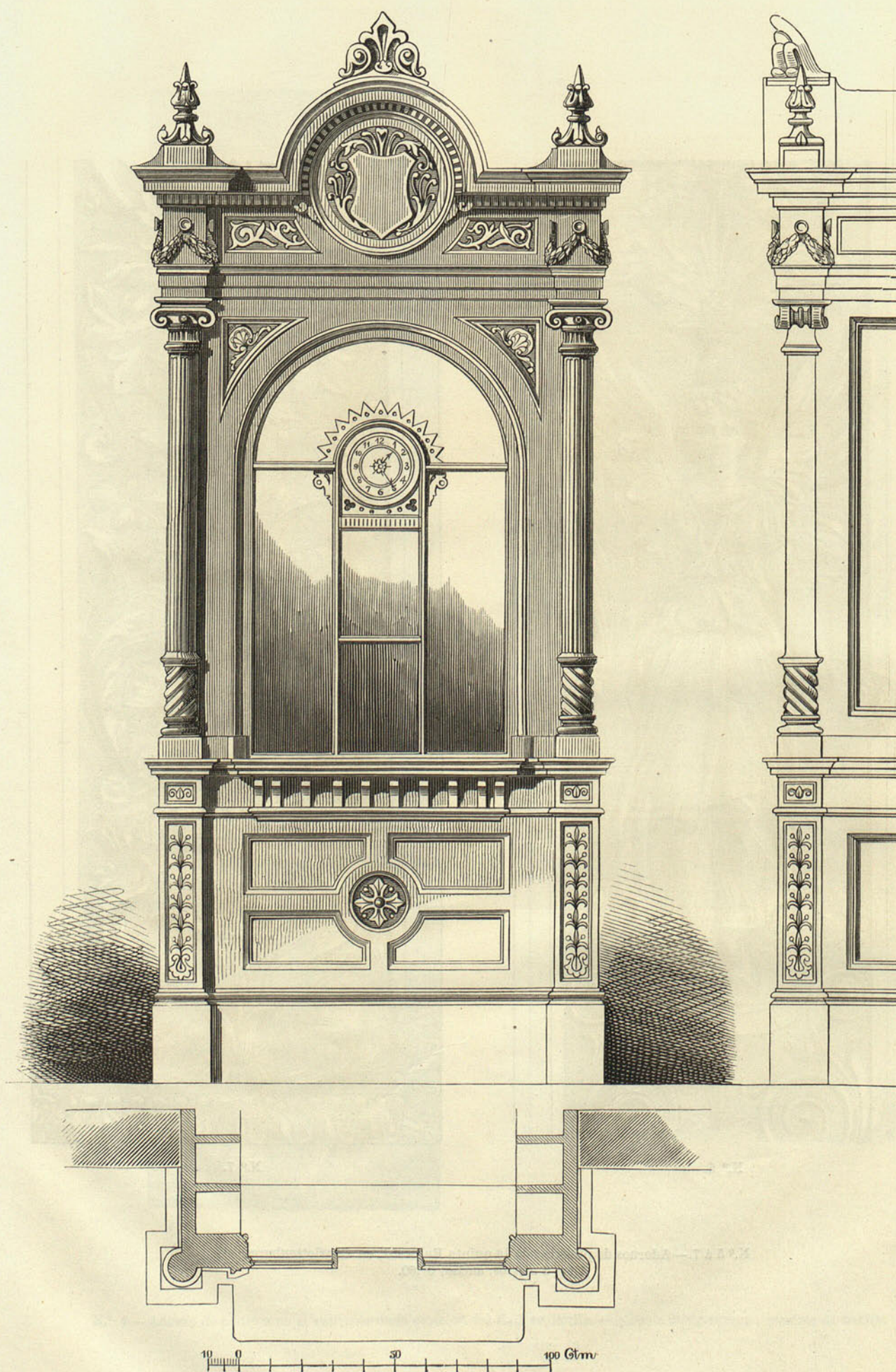
N.º 8 á 10. — Proyecto de despacho de billetes para una estacion de ferro-carril. — M. Wolanek, de Viena.
