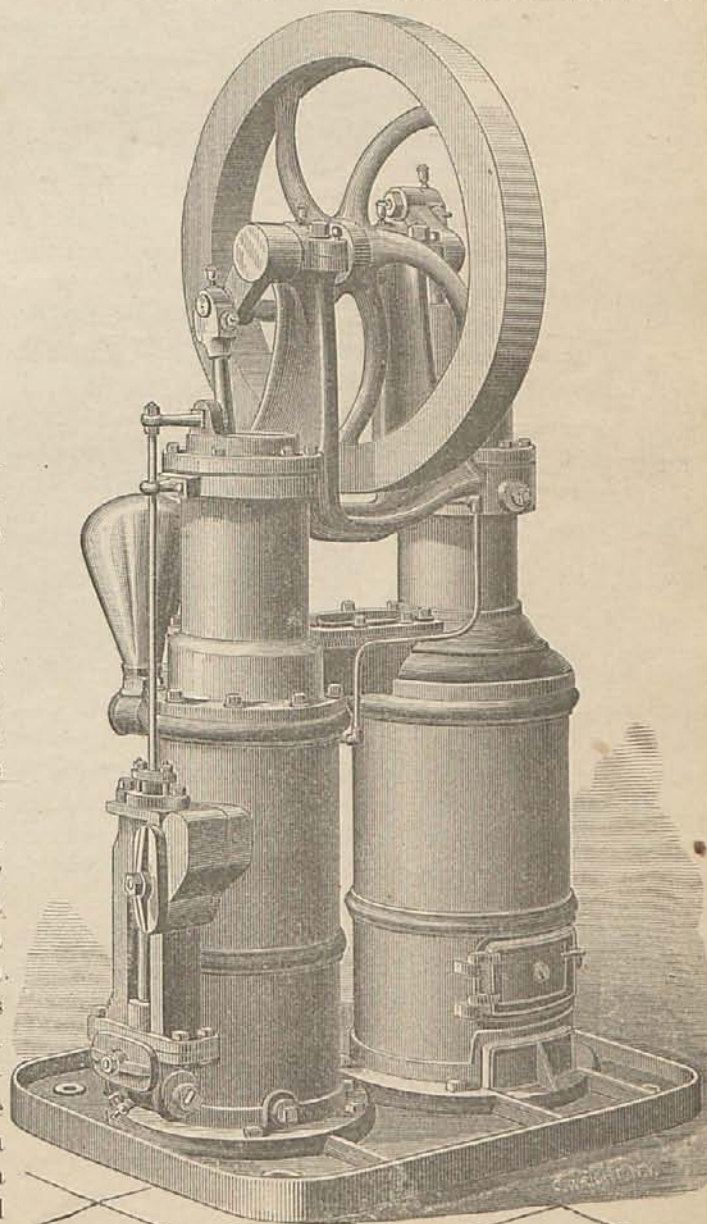
BOMBA CALÓRICA "RIDER."
