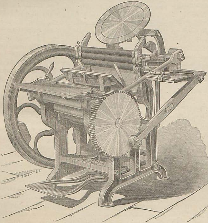
PRENSAS DE GORDON.
