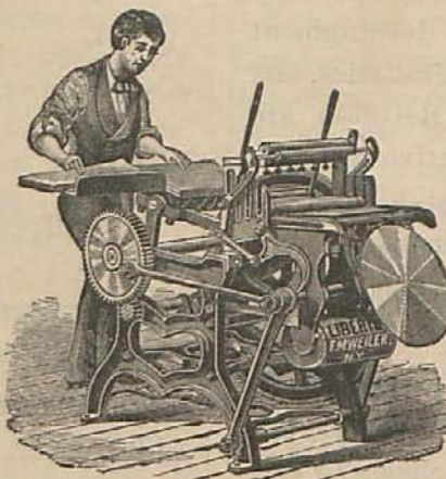
Prensa de Rotacion Liberty.
