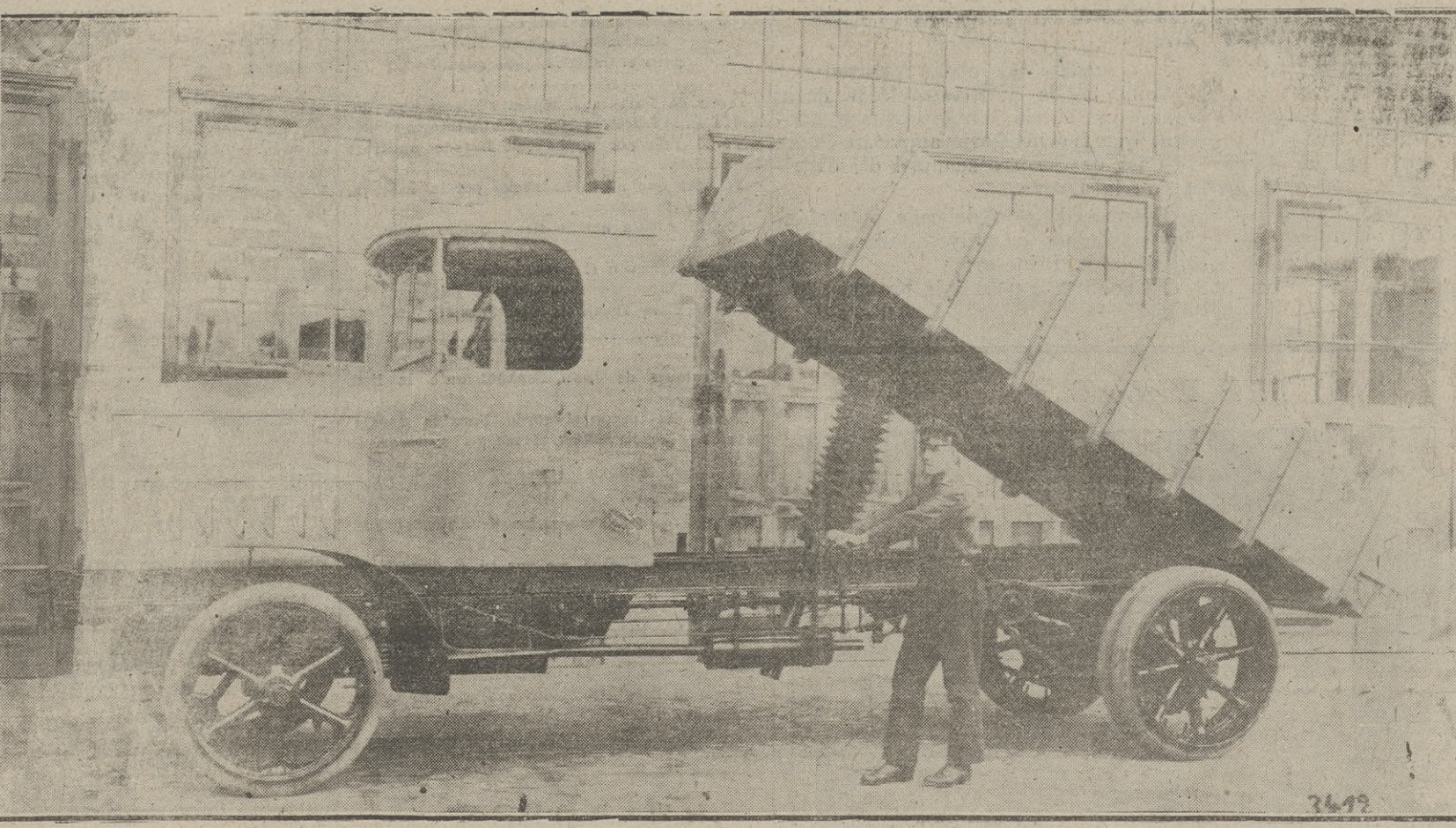
Camión-automóvil de cinco toneladas. 40 caballos. Modelo original «BUSSING», con perfeccionamientos e innovaciones técnicas protegidas por patentes
