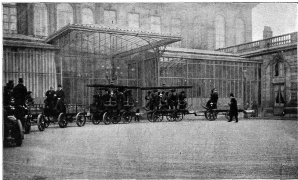
PARÍS. — El tren sin carriles del coronel Renard dispuesto para los viajes de ensayo, en el patio de sus locales de la calle de la Federación.
