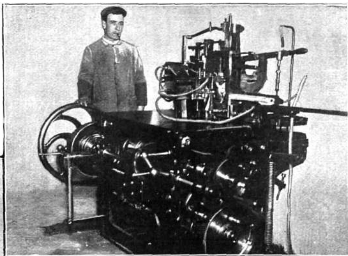
Modelo de máquina Foucher, que funde tipo desde el cuerpo 40 hasta los más grandes. Reune, á las demás ventajas de las otras, la de producir todos los tipos con un puente en su base perfectamente acabado, que reduce su peso, da más solidez á la letra y es de más cómodo empleo.
