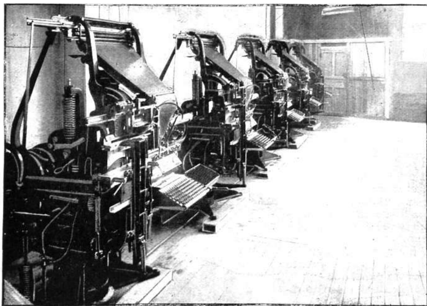
Una instalación de máquinas «Linotype» en disposición de funcionar.
