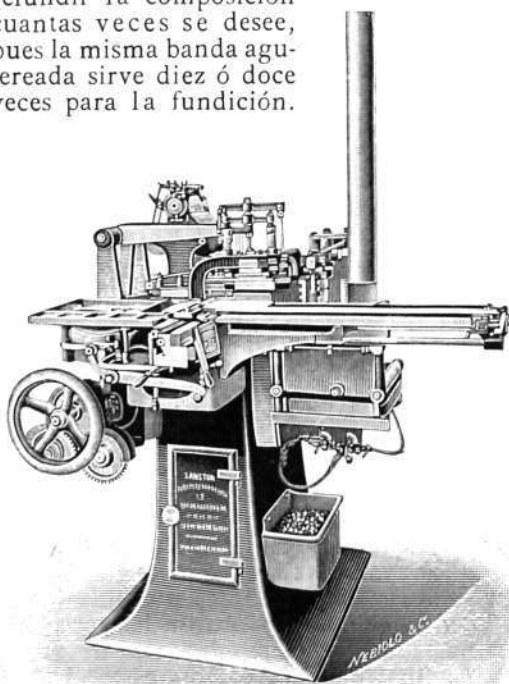
Máquina norte-americana sistema «Monotype.»
