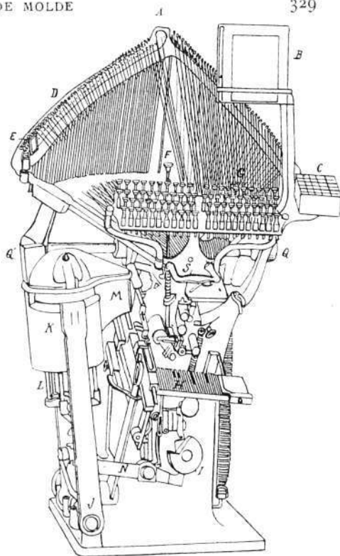
Pertil de la máquina alemana de componer sistema «Typograph».
