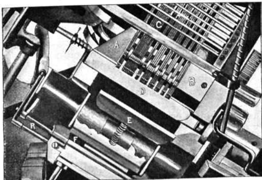
Línea compuesta en la máquina «Typograph» en el instante de ajustarse el molde.
