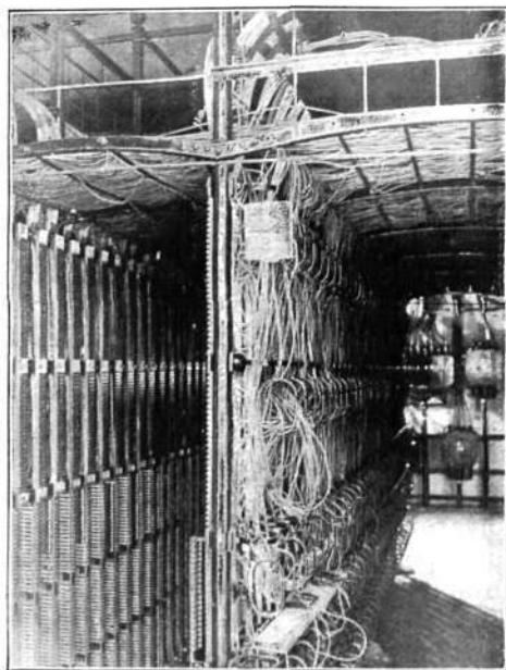
FIG. 3. Subterráneo en donde convergen los cables eléctricos que llegan del exterior para ser dirigidos desde allí á la cámara de distribución.
