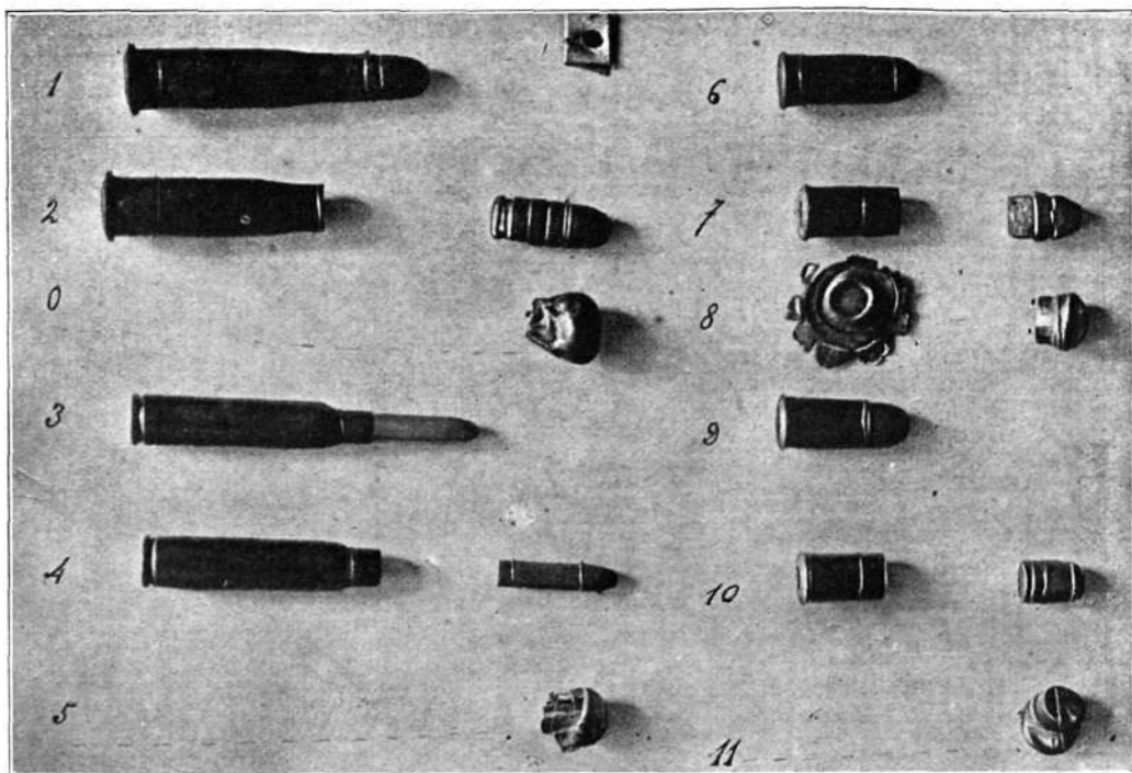
Núms. 1 a 5. Balas de fusil de reglamento antes y después de disparar contra la coraza.
