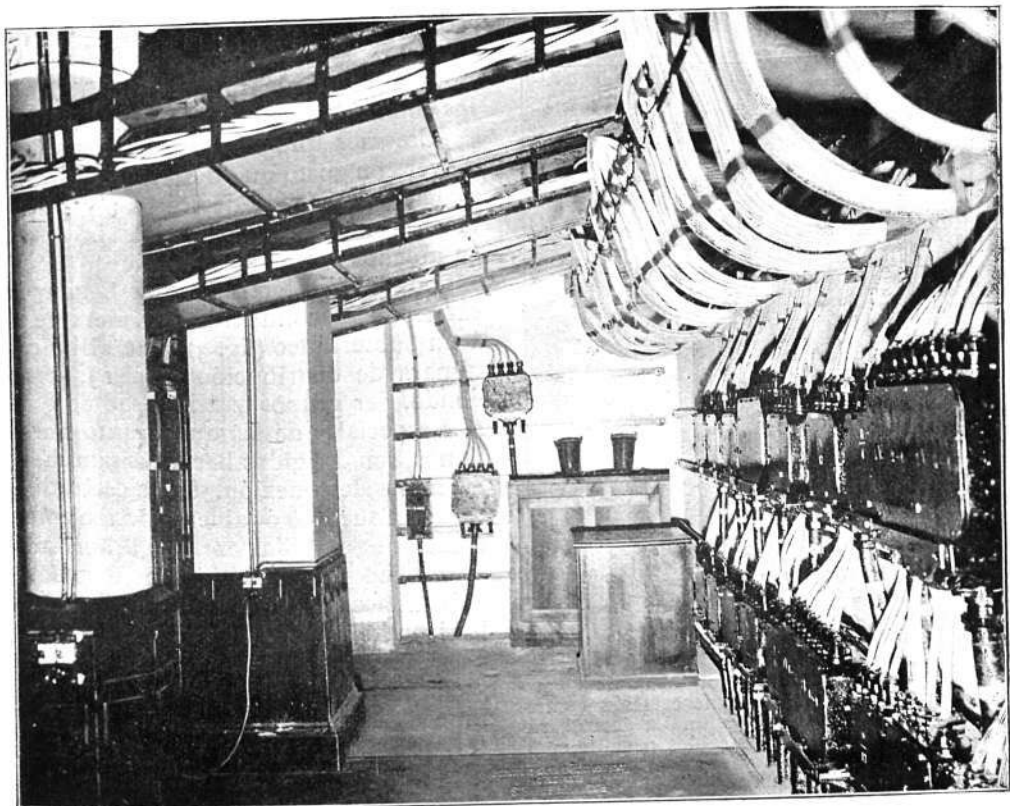
FIG. 1. Cámara de distribución, desde donde, por grupos, van los cables eléctricos hasta las mesas de comunicación en que prestan servicio las señoritas telefonistas.
