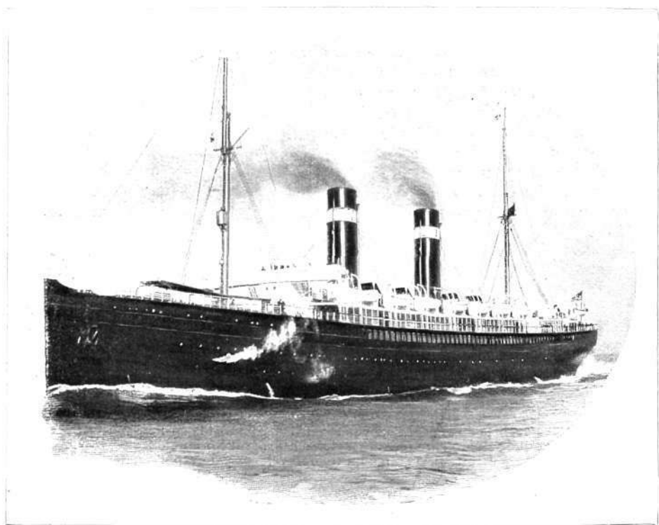
El vapor Saint-Paul , de la Compañía Americana, construido en 1894 en Filadelfia. Desaloja 11.629 toneladas, tienen sus máquinas una fuerza de 20.000 caballos y mide 60 metros de eslora.
