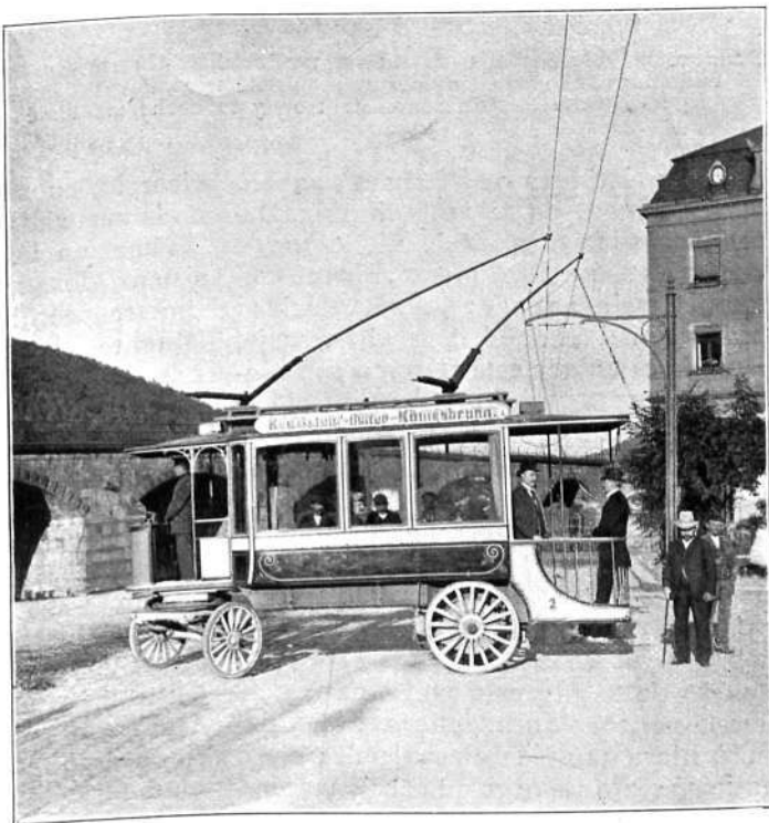
Omnibus eléctrico de la compañía Siemens-Halske, que recorrió en sus primeras pruebas un trayecto de veintiún kilómetros desde el fondo del valle de Biela hasta la estación de Königstein, con velocidad de doce kilómetros por hora. El contacto se establecía por medio de dos troles.
