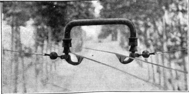
Pieza de tubo de hierro, en forma de C, que sostiene los alambres sobre aisladores de porcelana. Esta disposición se emplea cuando la línea se halla en el centro del camino.
