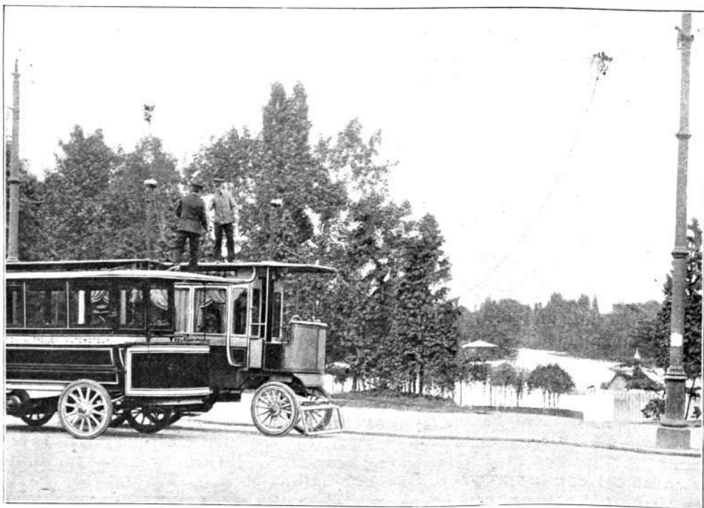
Omnibus movido por el trole auto-motor Lombard-Guerin. En este sistema el trole no es arrastrado por el carruaje, sino por un motor eléctrico. Por medio de un mecanismo automático se asegura la velocidad sincrónica del trole y del coche, manteniéndose el cable á la debida altura.
