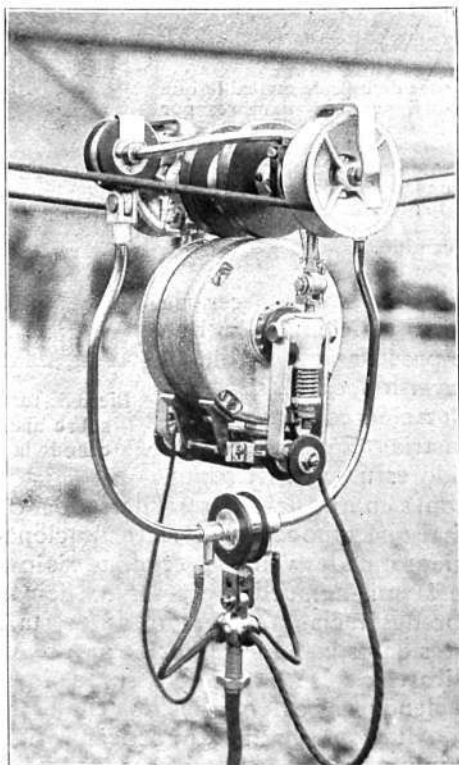
Motor trifásico del trole, susceptible de funcionar á tres velocidades distintas y actuar también en sentido de abajo arriba por medio del marco que sostiene el eje superior.
