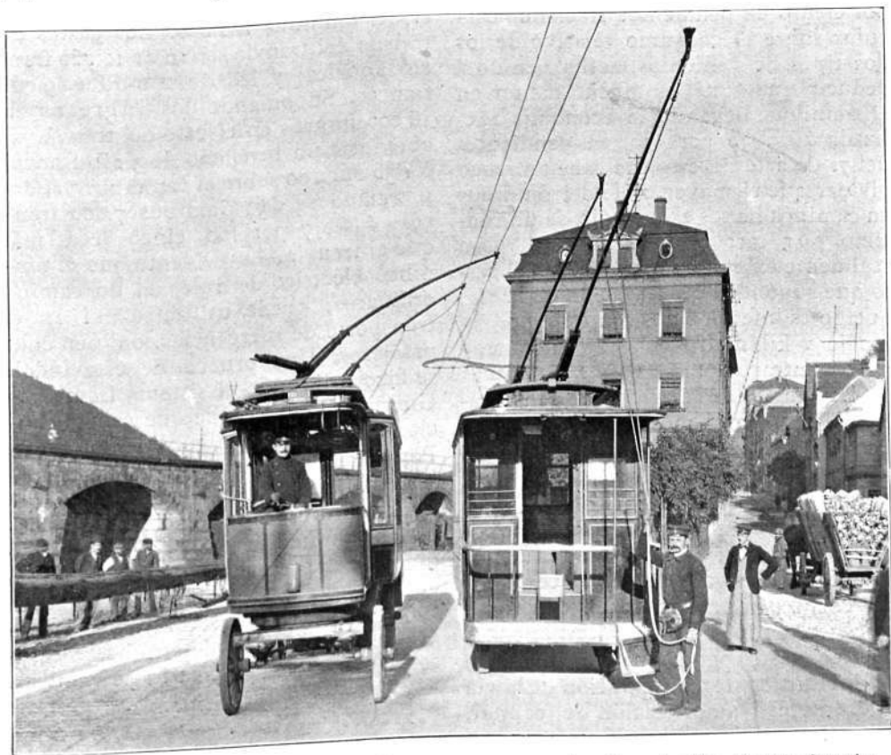
Dos ómnibus sistema Siemens-Halske al cruzarse en su camino. Uno de ellos, el de la derecha, detiéndose y baja sus troles mientras el otro continúa la marcha.
