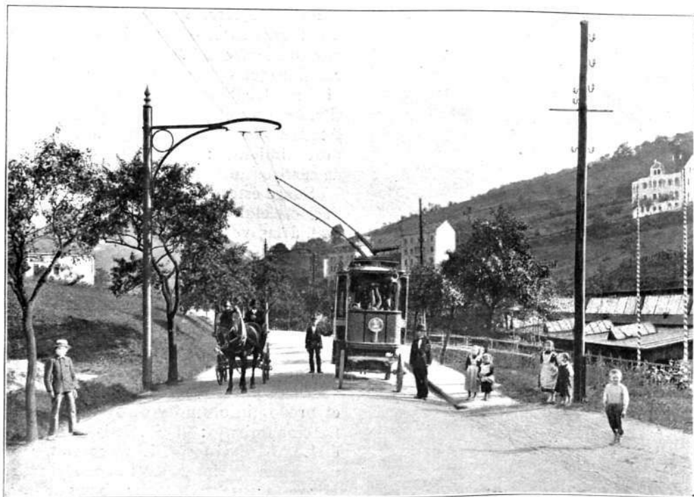
Tranvía sin carriles ú ómnibus eléctrico en el momento de evitar el choque con uno de los carruajes que transitan por la vía pública.
