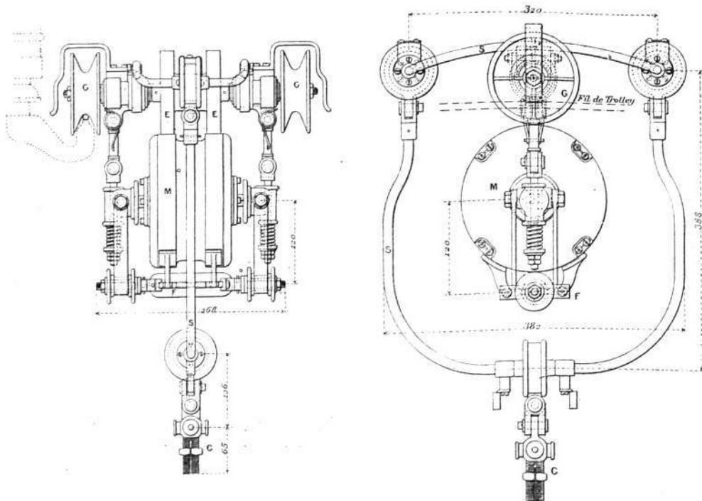
Dibujo esquemático del trole auto-motor Lombard-Guerin. Es de aluminio y su peso no excede de veinte kilogramos.
