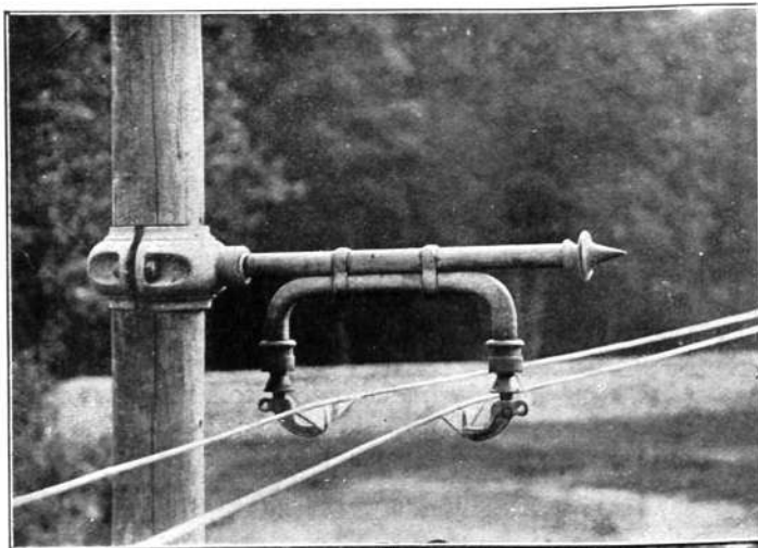
Postes de bronce maleable que sostienen los alambres por donde circula la corriente. Los aisladores de porcelana van fijos en la pieza inferior, que tiene forma de C. Esta disposición se emplea cuando la línea está á un lado del camino.
