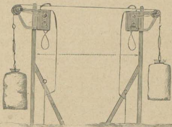
FIG. 1.ª—Sistema telefónico militar de M. Charollois.
