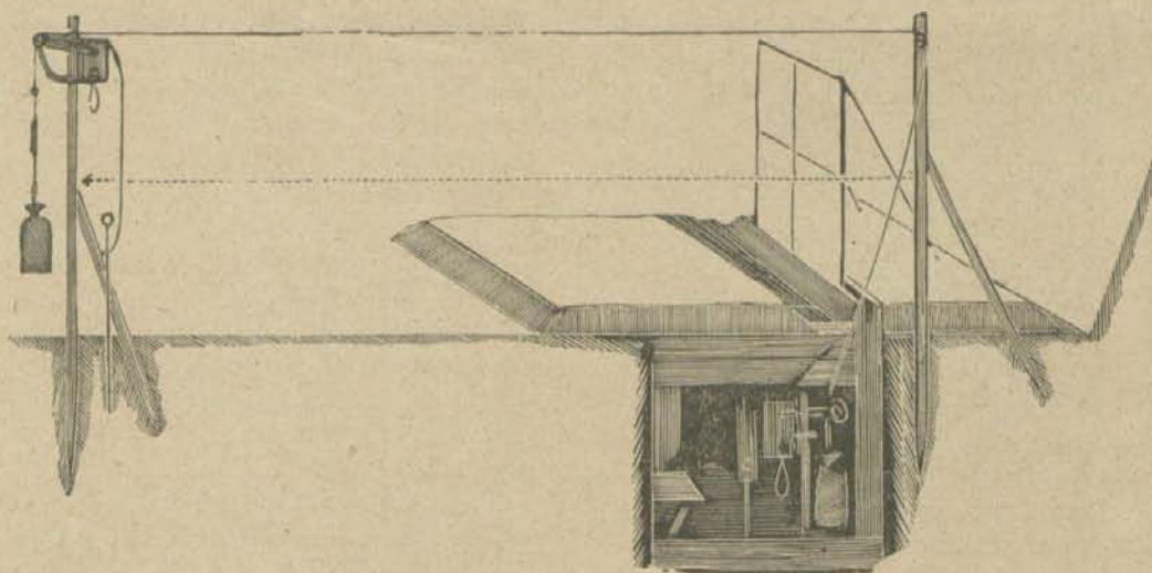
FIG. 2.ª—Montaje del sistema telefónico militar de M. Charollois en un campo de tiro.
