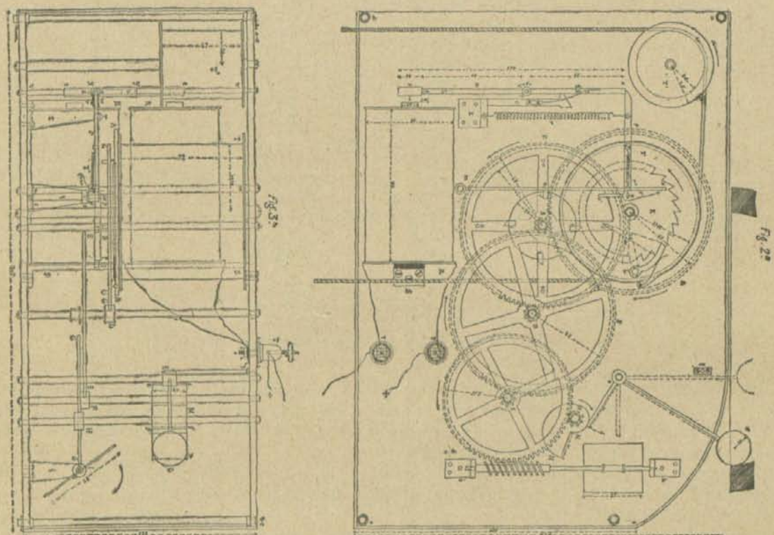
VI.—Aparato electro-mecánico para los pasos a nivel.
