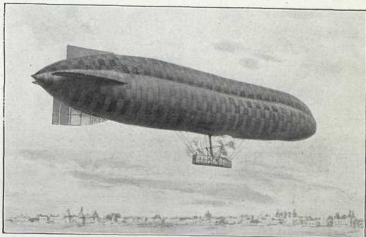
Dirigible inglés Astra Torres XIV , flexible, de 8,700 m. 2 ; longitud, 77 m.; diámetro, 18 m.; motores, 400 H. P.; velocidad, 82'2 kilóm. Construido en 1913
