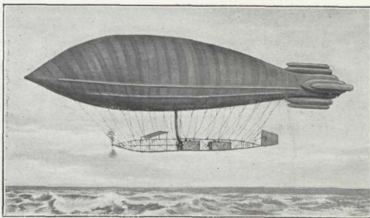
Dirigible francés Ville de Paris , flexible, de 3,200 m. 2 ; longitud, 60'4 m.; diámetro, 10'5 m.; motores, 70 H. P.; velocidad, 43'2 kilóm. Construido en 1903
