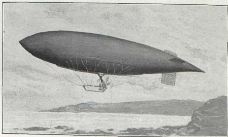
Dirigible inglés Parseval , flexible, de 8,800 m. 2 ; longitud, 84 m.; diámetro, 15 m.; motores, 360 H. P.; velocidad, 68 kilóm. Construido en 1913
