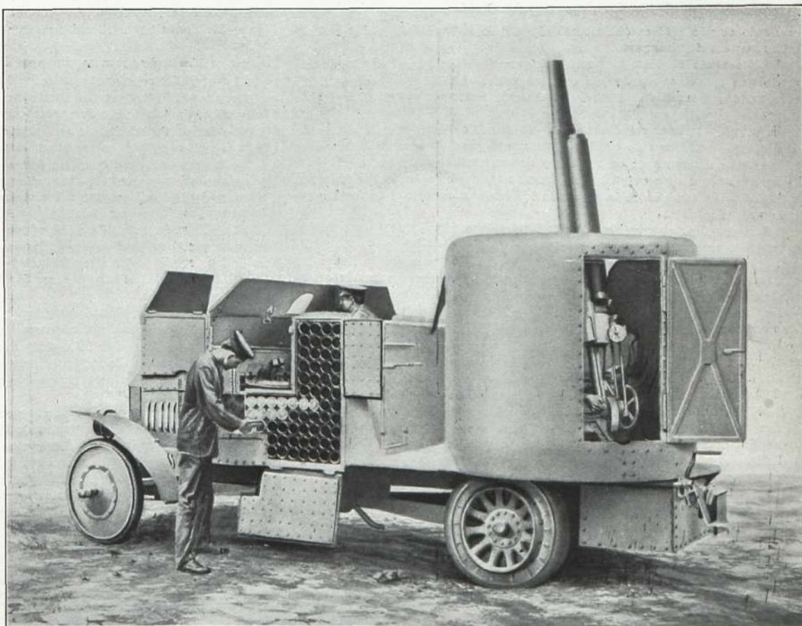
Cañón del ejército alemán, de 71 mm., contra aeroplanos y dirigibles, montado en un automóvil blindado
