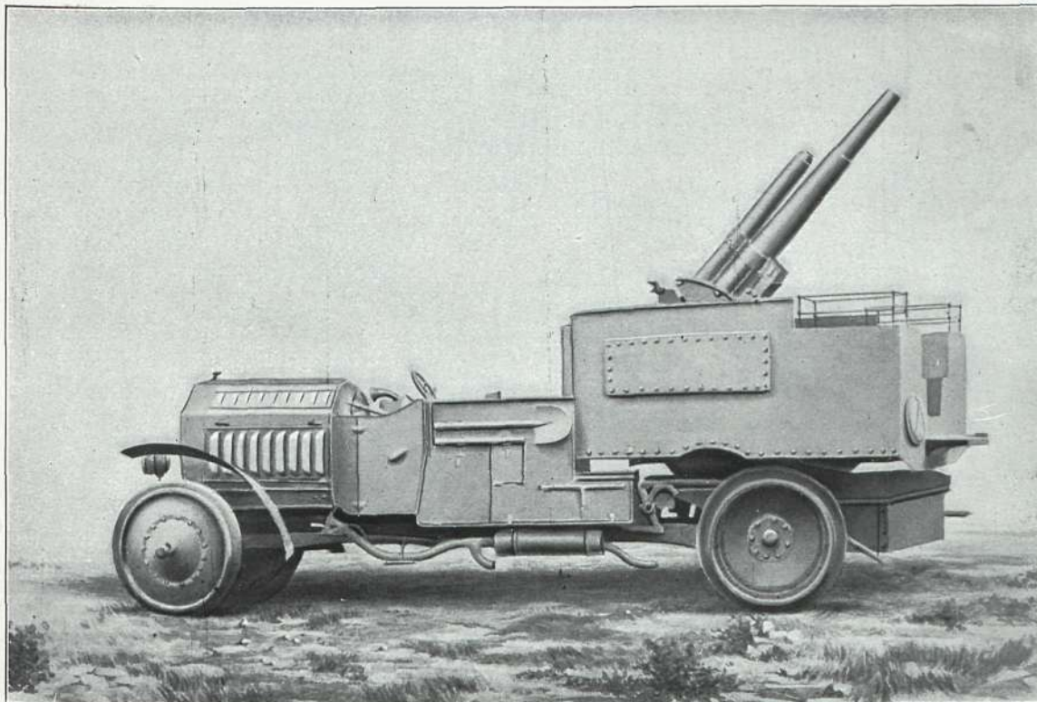
Cañón del ejército alemán, de 71 mm., contra aeroplanos y dirigibles, montado en un automóvil
