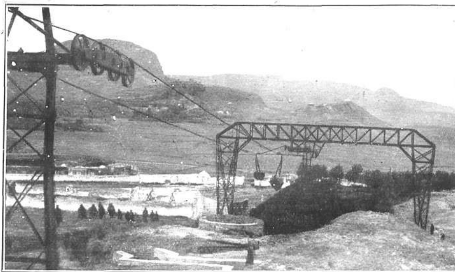
Descargadores de mineral en San Juan de las Minas.
