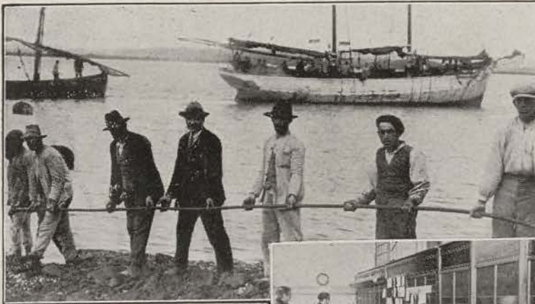
Arriba: Obreros españoles tendiendo el cable telefónico de Ayamonte (Huelva) a Villarreal de Santo Antonio (Portugal). A la derecha: Lisboa. Cuadro interurbano de la Central.
