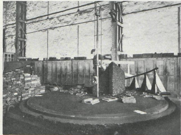
Figura 3.ª—Preparativos iniciales para el moldeo de una hélice de bronce manganeso
