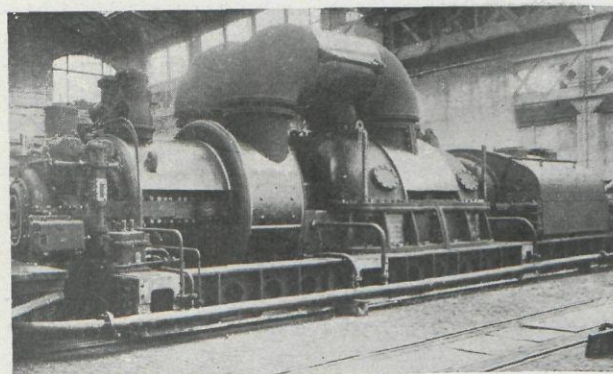
Figura 3.ª—Un grupo turbo-alternador. El buque lleva cuatro grupos análogos a éste, de 42.000 CV. cada uno
