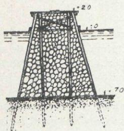
Figura 5.—Sección tipo del dique Norte.
