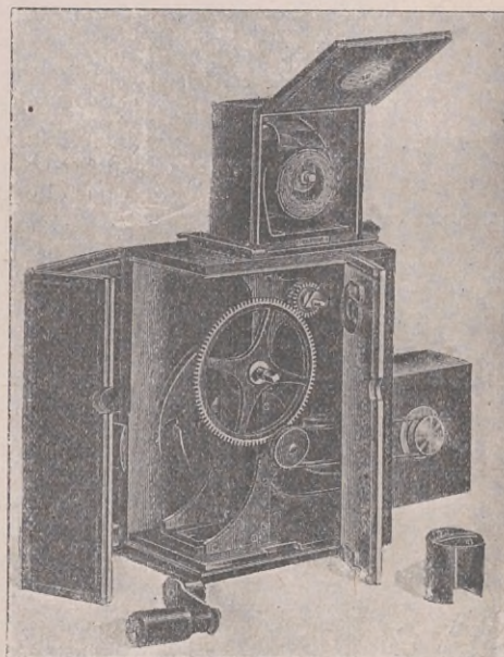
EL MIRÓGRAFO DISPUESTO PARA TOMAR UNA FOTOGRAFÍA
