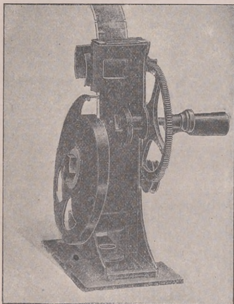
EL MIRÓGRAFO: MECANISMO DE ARRASTRE Y DE OBTURACIÓN
