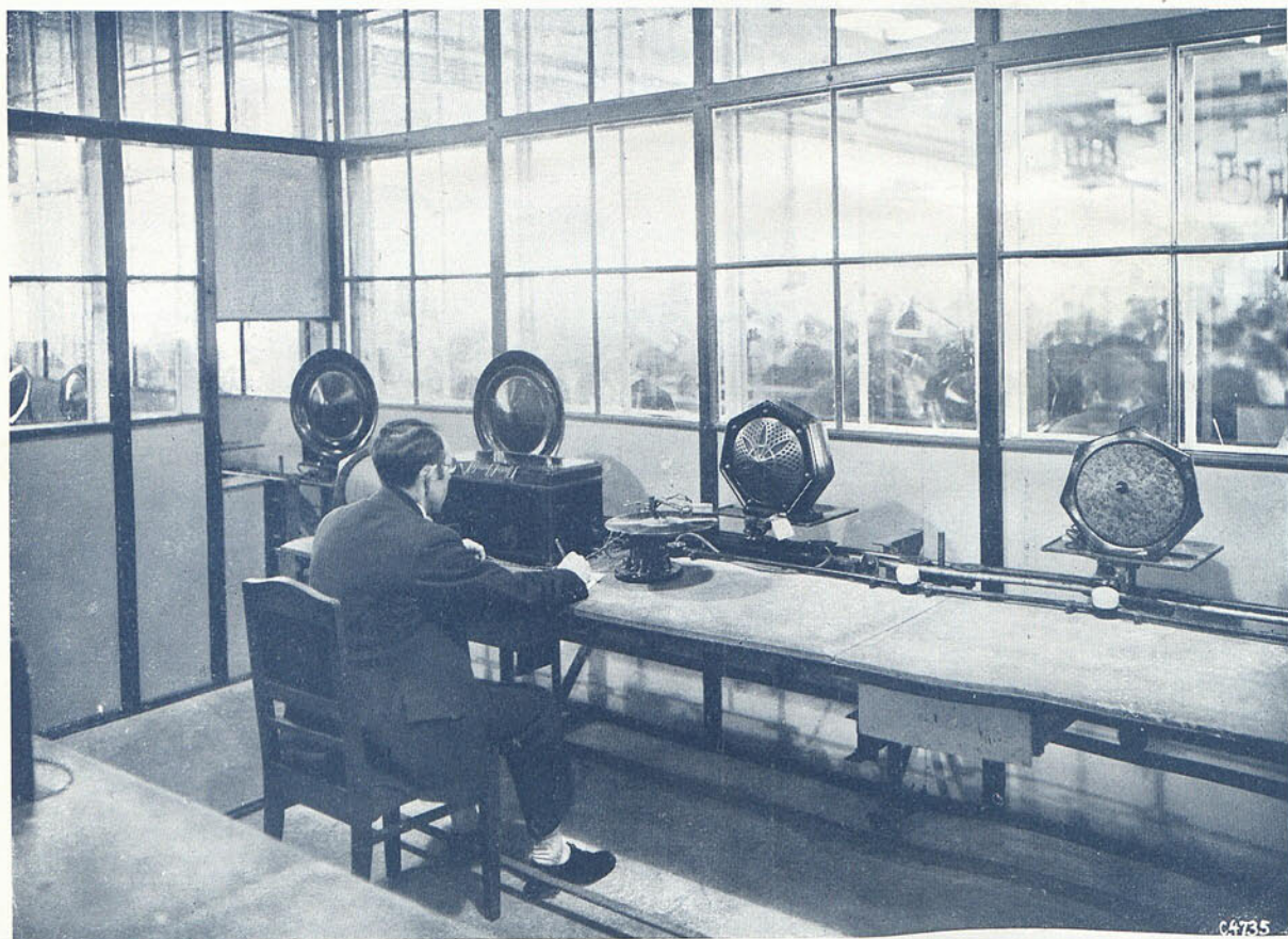
Una de las salas de comprobación. - Los altavoces pasan por correa sinfín, conectándose automáticamente a un receptor 2511 que actúa como amplificador fonográfico.
