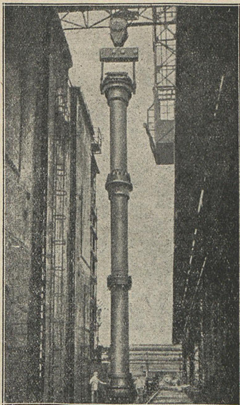
Un catalizador en el cual se efectúa la síntesis del amoniaco. El amoniaco es fabricado en estos aparatos por contacto del hidrógeno y del ázoe, a 200 atmósferas en presencia del óxido de hierro.
